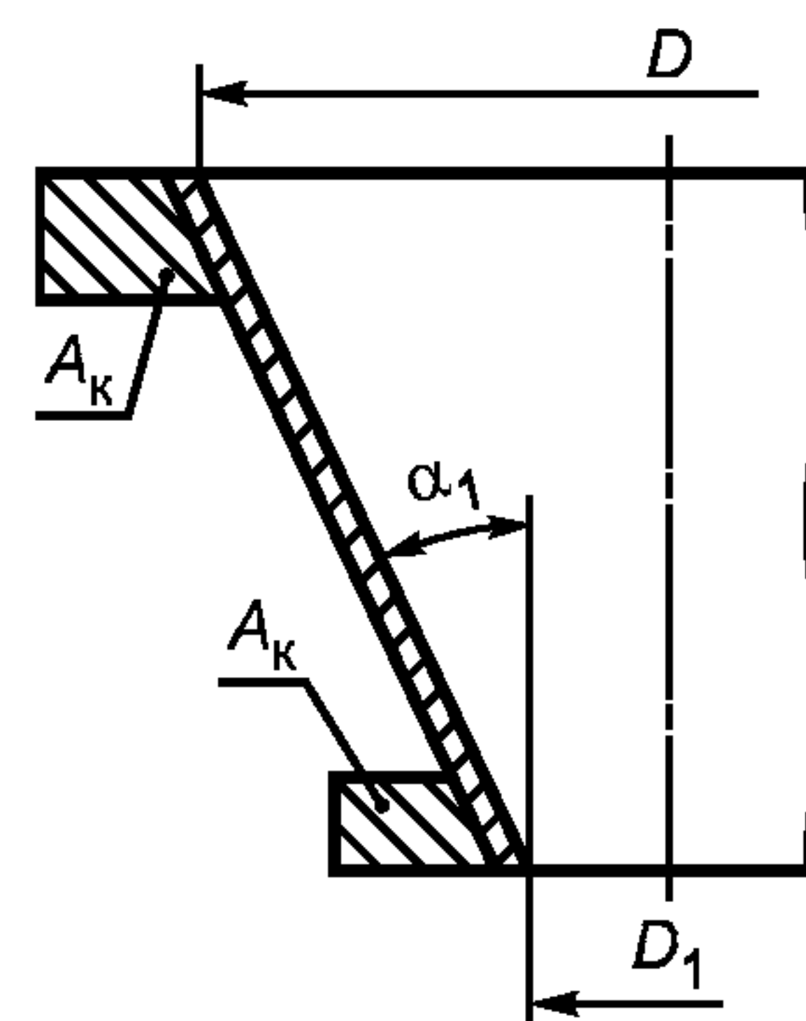
Рисунок 29 — Коническая обечайка с кольцами жесткости
