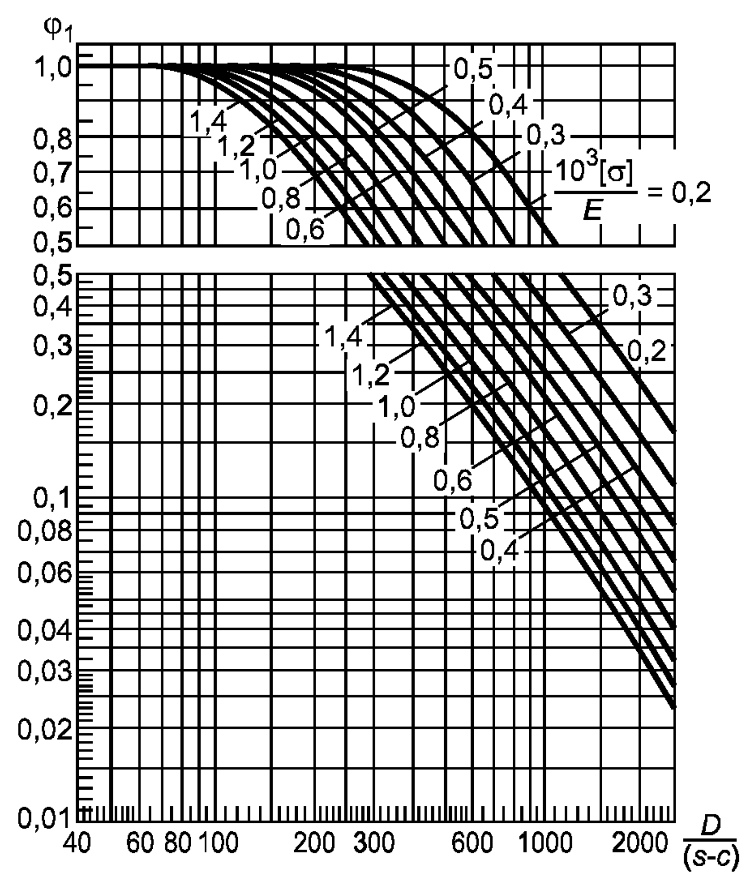
Рисунок 5 — График для определения коэффициента \phi_1
