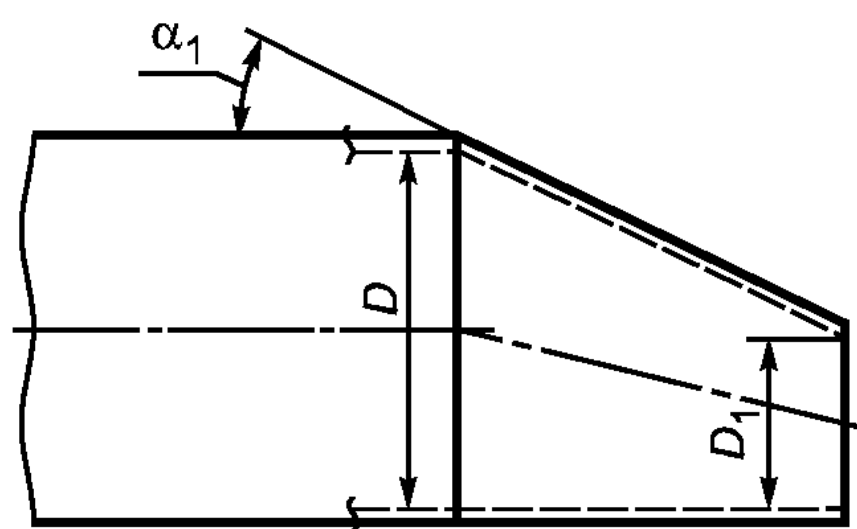
Рисунок 28 — Соединение кососимметричных обечайек
