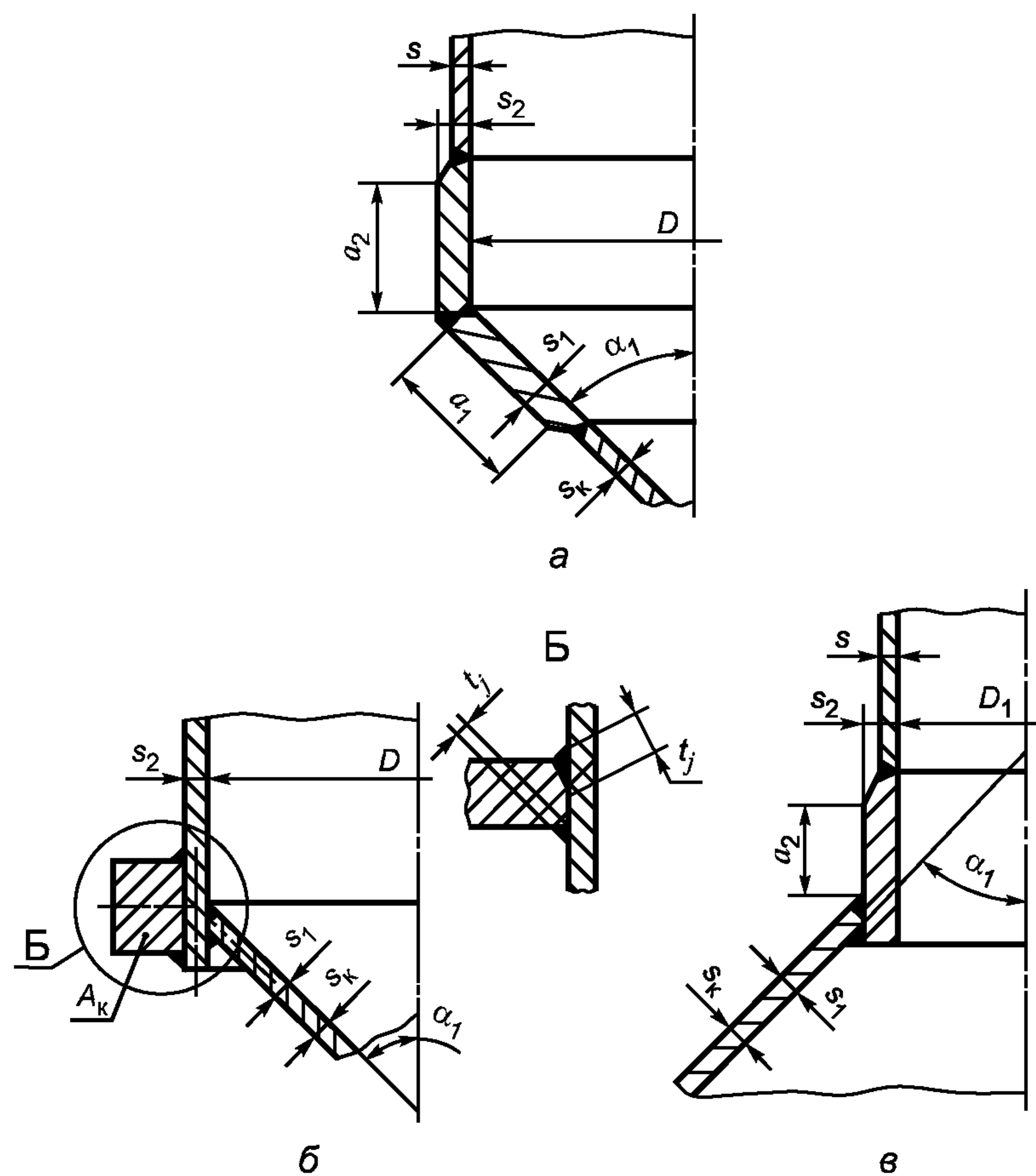
а — соединение конической и цилиндрической обечаек, б — соединение конической и цилиндрической обечаек с укрепляющим кольцом, в — соединение конической обечайки с цилиндрической меньшего диаметра
