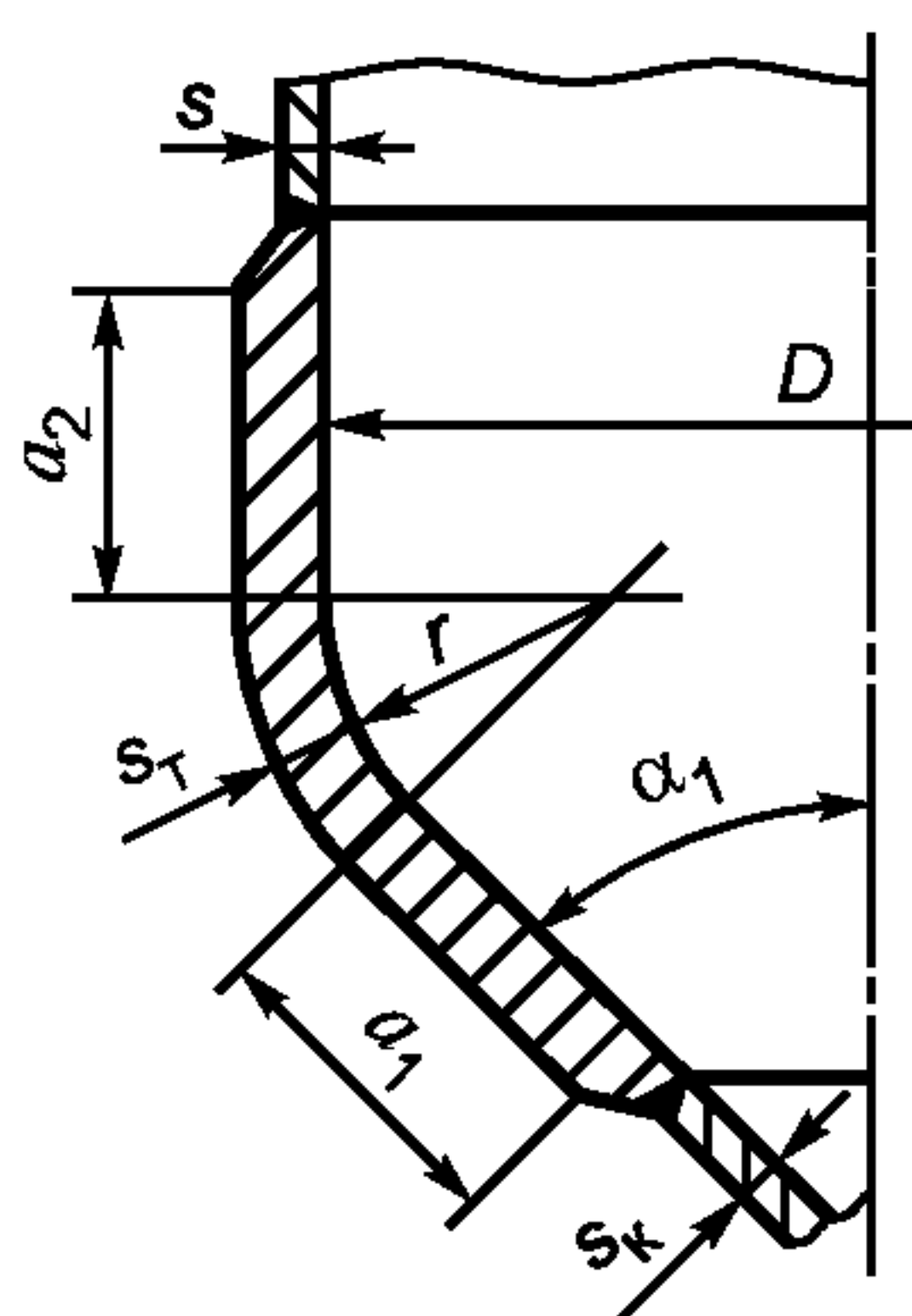
Рисунок 26 — Соединение обечайек с тороидальным переходом
