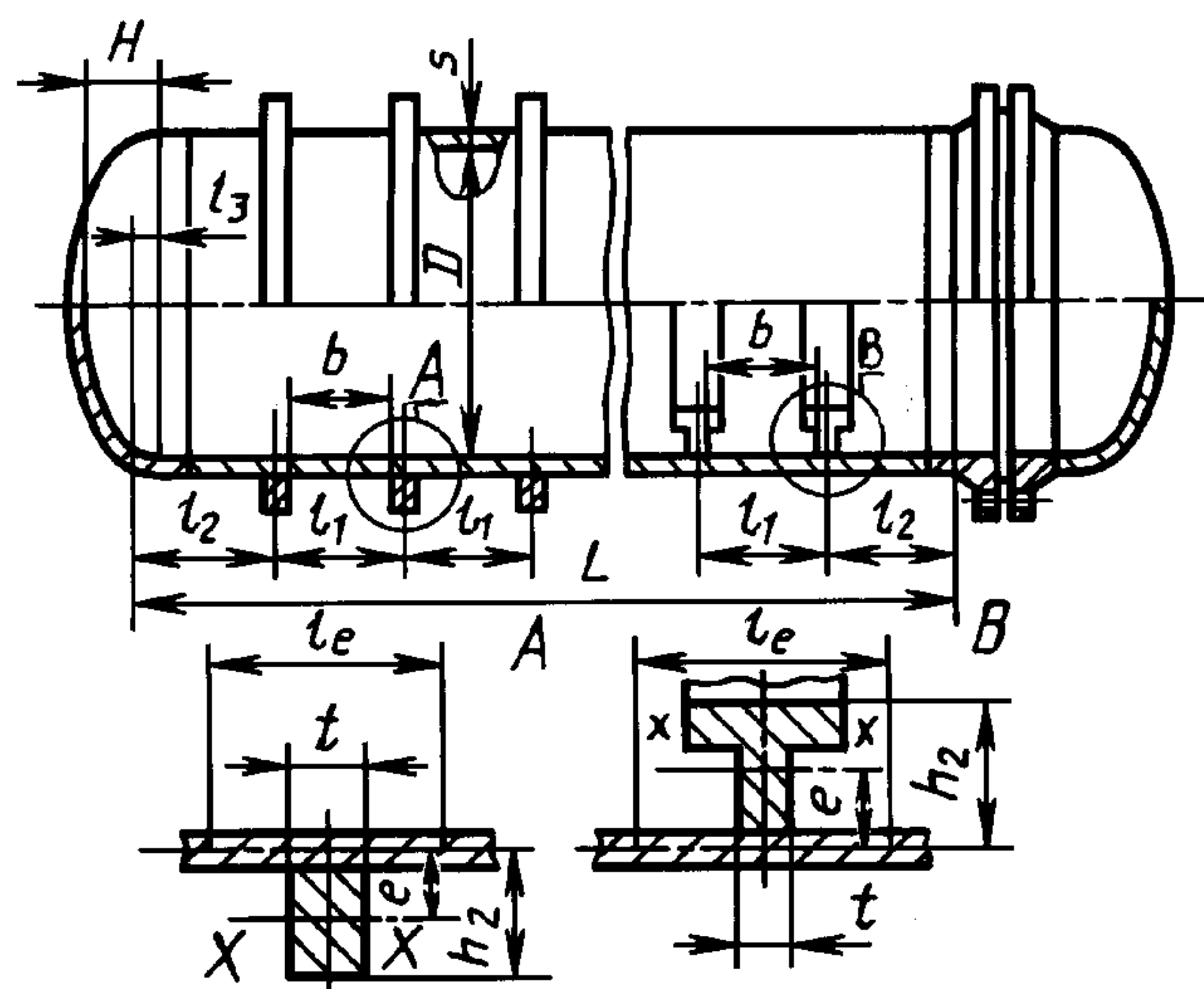
Рисунок 4 — Цилиндрическая обечайка, подкреплённая кольцами жесткости
