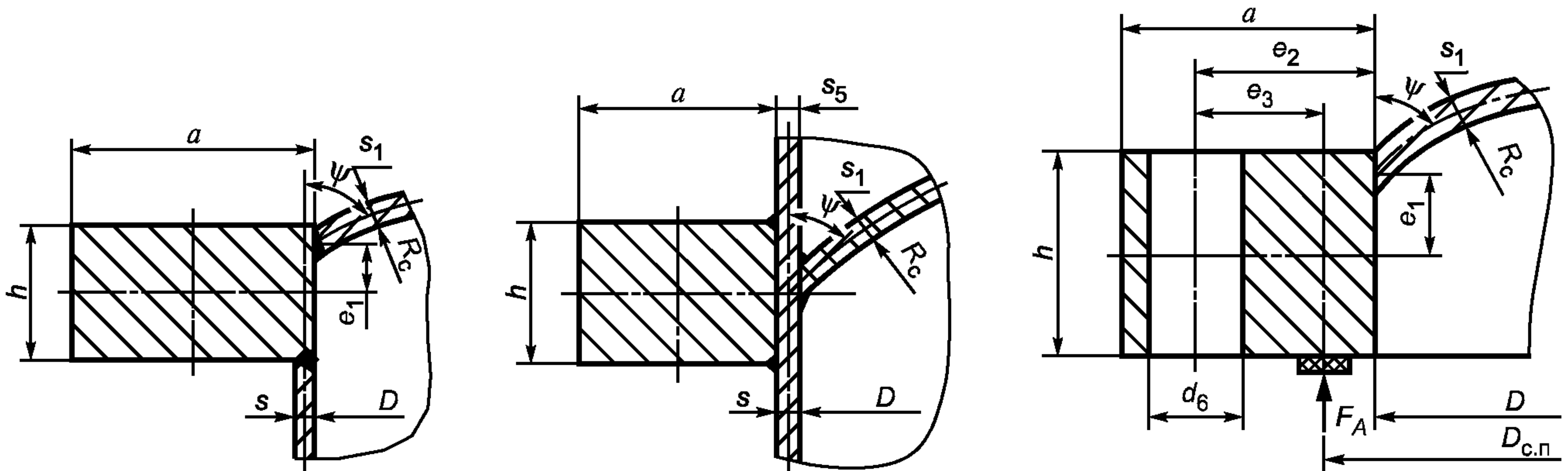
Рисунок 13 — Сферическое неотбортованное днище с укрепляющим кольцом
