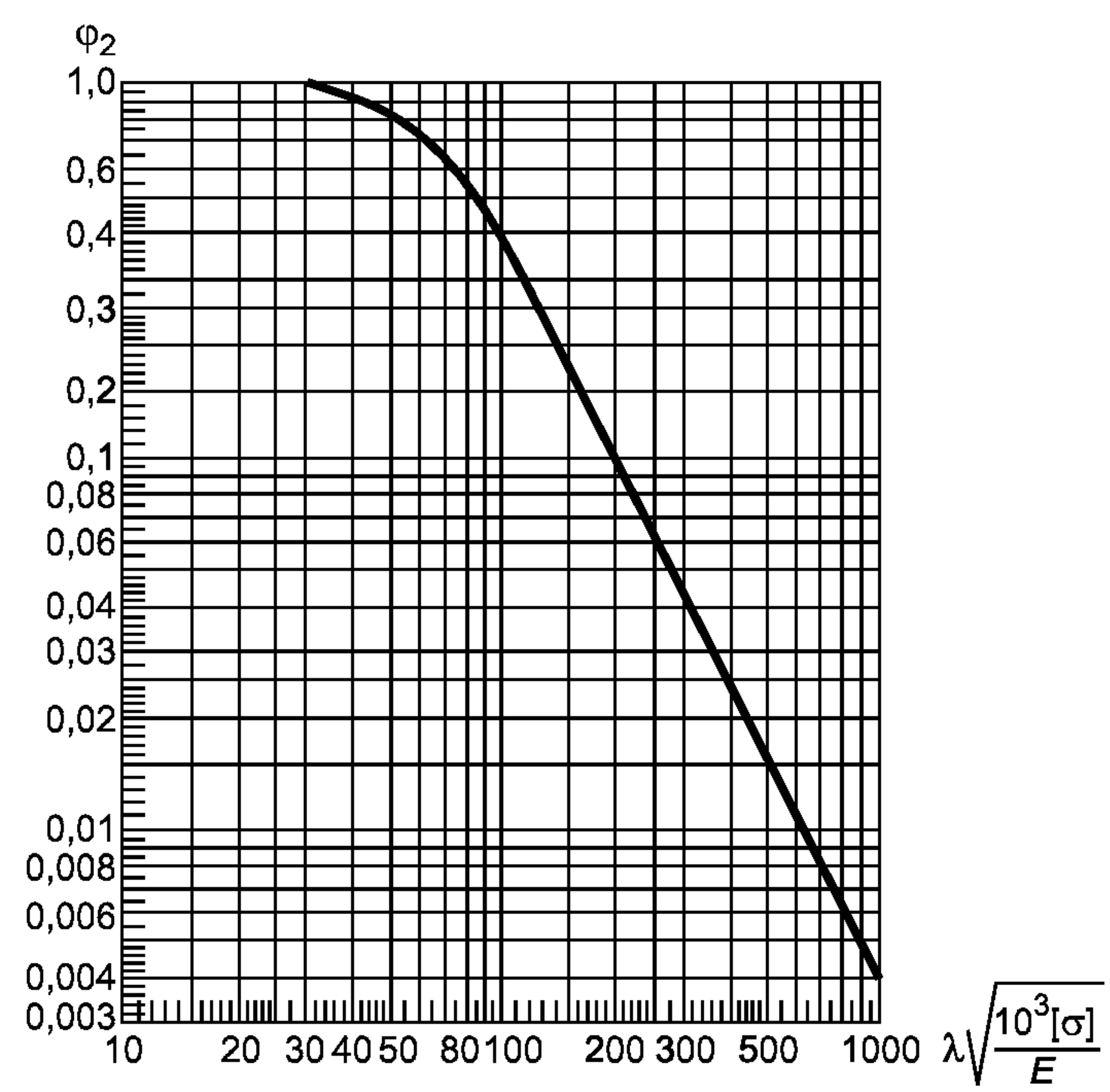
Рисунок 6 — График для определения коэффициента \phi_2
